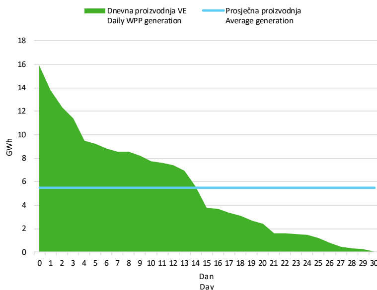
Slika 6 Krivulja trajanja dnevne proizvodnje vjetroelektrana u listopadu 2024. godine
