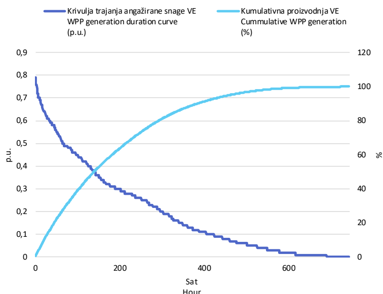
Slika 3 Krivulja trajanja angažirane snage svih VE i kumulativna proizvodnja VE u listopadu 2024. godine u jediničnim vrijednostima
