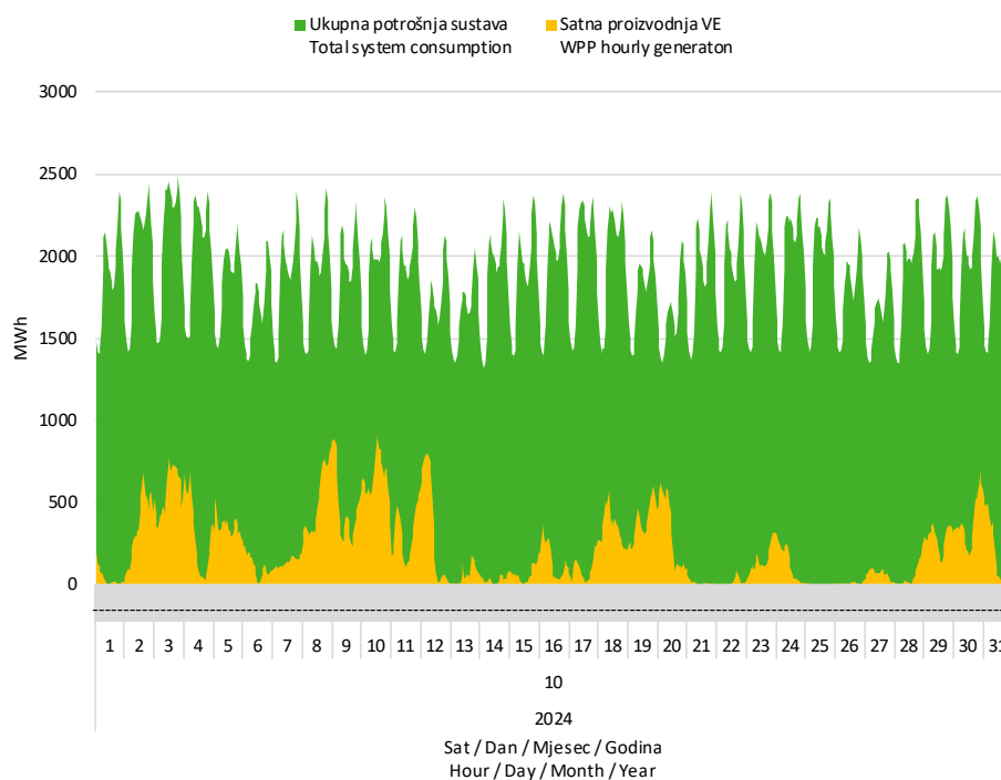
Slika 7 Usporedba satnog dijagrama opterećenja sustava i proizvodnje vjetroelektrana u listopadu 2024. godine
