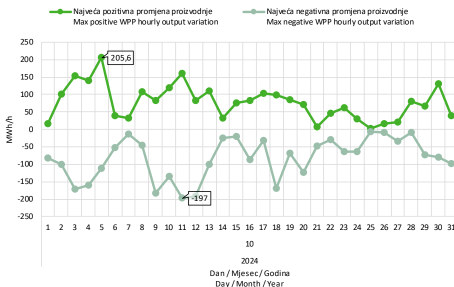
Slika 9 Maksimalna pozitivna i maksimalna negativna promjena satne proizvodnje VE u listopadu 2024. godine
