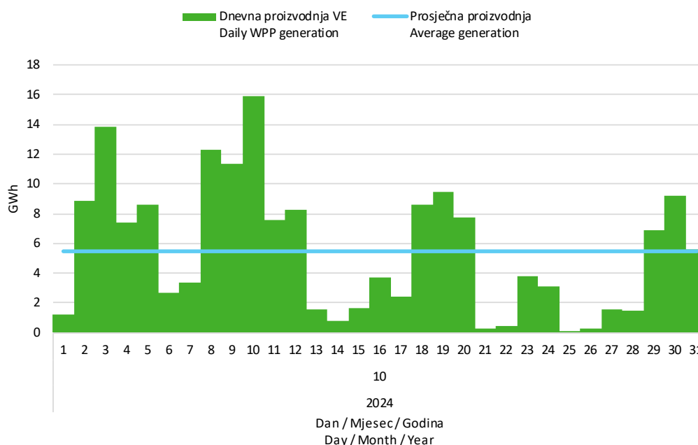
Slika 5 Dnevna proizvodnja svih vjetroelektrana u listopadu 2024. godine
