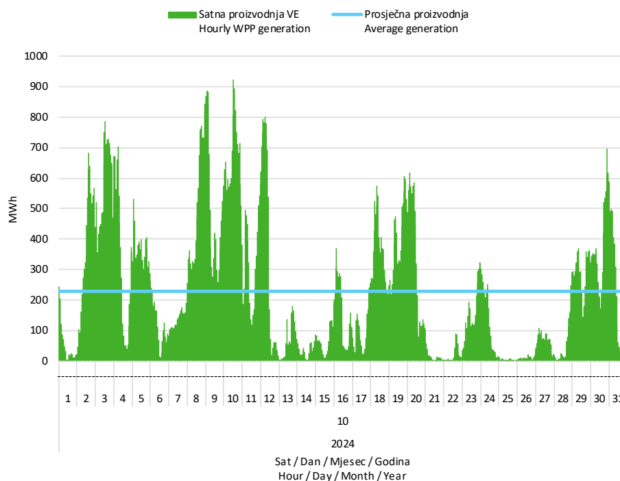
Slika 2 Satna proizvodnja svih vjetroelektrana u listopadu 2024. godine
