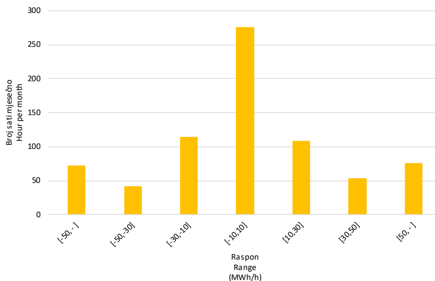
Slika 10 Statistička raspodjela satnih promjena proizvodnje VE u listopadu 2024. godine
