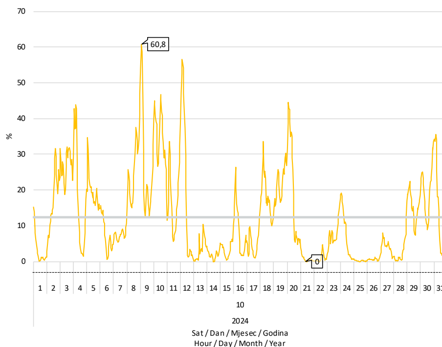
Slika 8 Udio proizvodnje vjetroelektrana u pokrivanju satnog opterećenja elektroenergetskog sustava u listopadu 2024. godine
